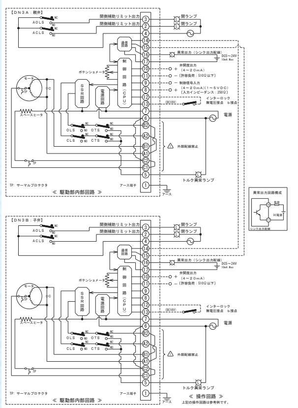
DN3 (3方弁比例制御)
