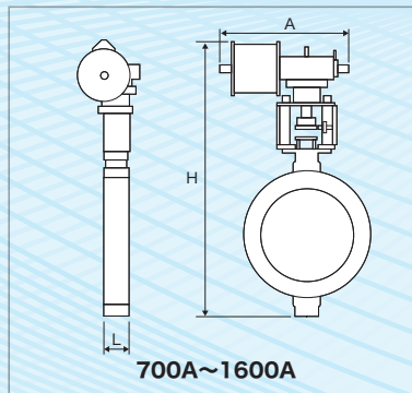
700A~1600A (単位 寸法 mm、質量 kg)
