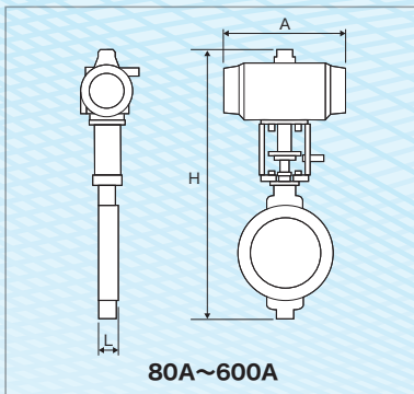
80A~600A (単位 寸法 mm、質量 kg)
