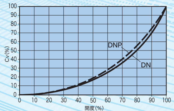
Cv値(開度グラフ)
