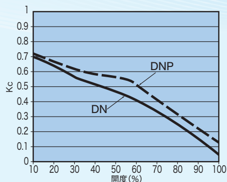
キャビテーション係数(Kc値)
