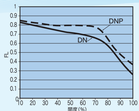
圧力回復係数(FL値)
